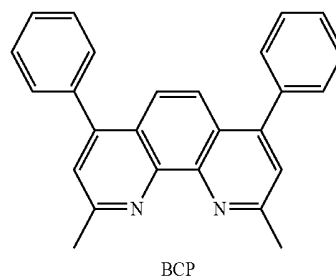
BCP
