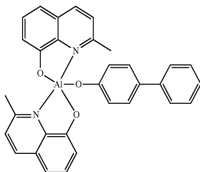
Balq
